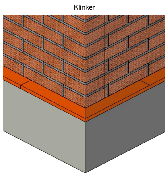
Рис. 22. Устройство внешних углов при помощи угловых элементов.
