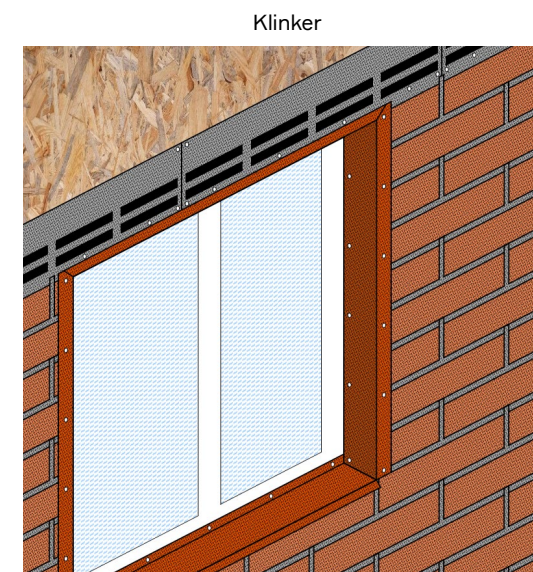
Рис. 28. Монтаж фасадной плитки над оконным проёмом.
